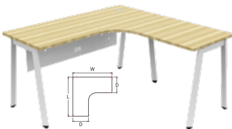
L-SHAPE TABLE
