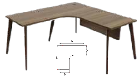
L-SHAPE TABLE
